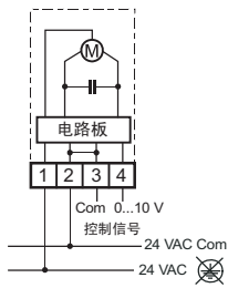
VA-7312接线图 (比例控制型)
