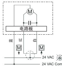
VA-7310接线图 (浮点控制型)
